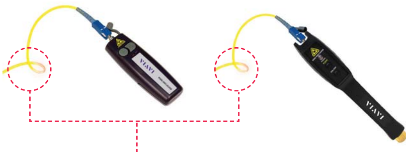
光ファイバの損傷箇所から漏出する赤色レーザー光
