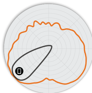
図 5. R550 5GHz エレベーションアンテナ パターン
