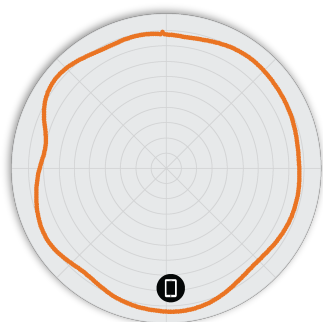
図 2. R550 2.4GHz アジマスアンテナ パターン
